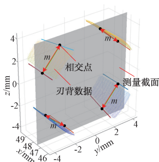
图 11 螺尖丝锥刃背宽度计算示意图
