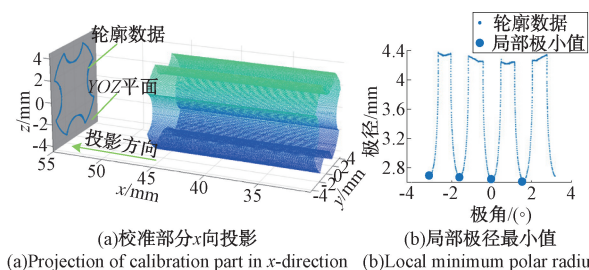
图8 螺尖丝锥芯径计算示意图
