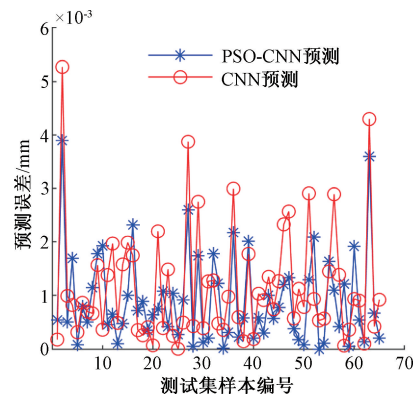
图 15 PSO-CNN 与 CNN 预测效果
