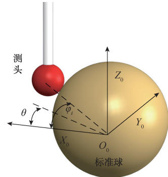
图7 测头校准示意图
