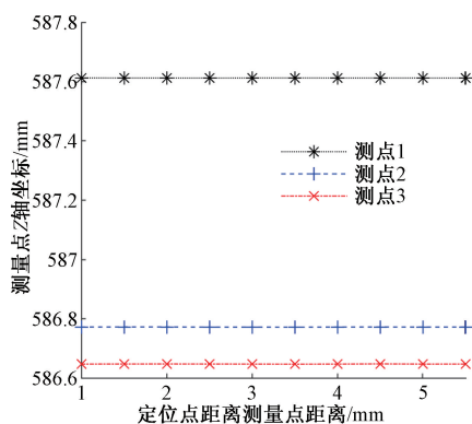
(a) 定位点对预行程误差影响
