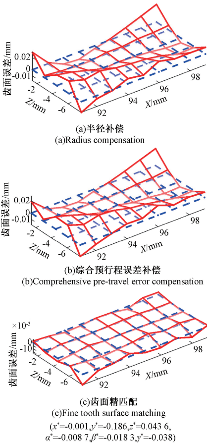
图 17 右齿面误差对比实验图
