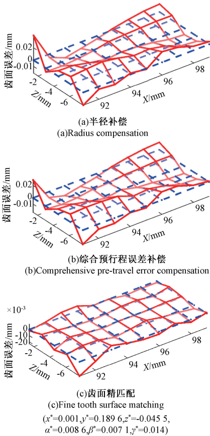
图 16 左齿面误差对比实验图
