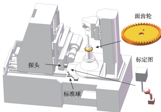
图 5 磨齿机模型图
