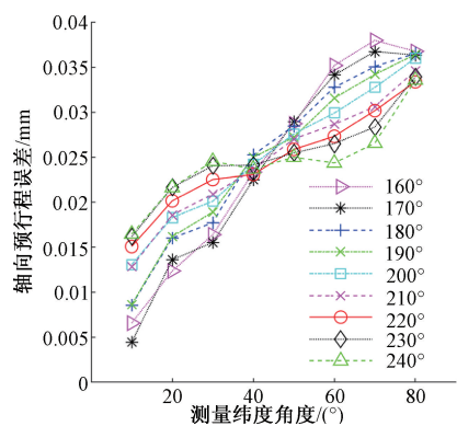
图 14 轴向预行程误差变化图
