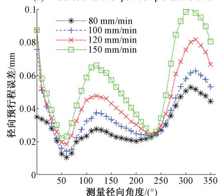
(b) 不同速度对径向预行程误差影响
