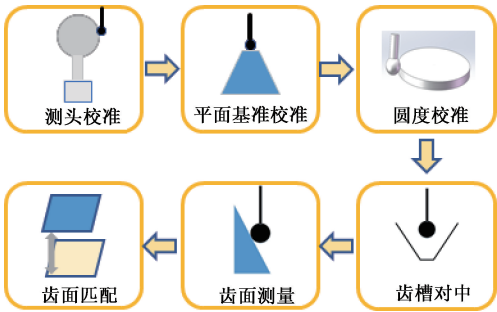
图 3 面齿轮在机测量流程图
