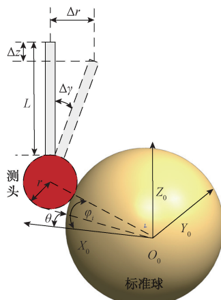
图9 轴向位置偏移示意图
