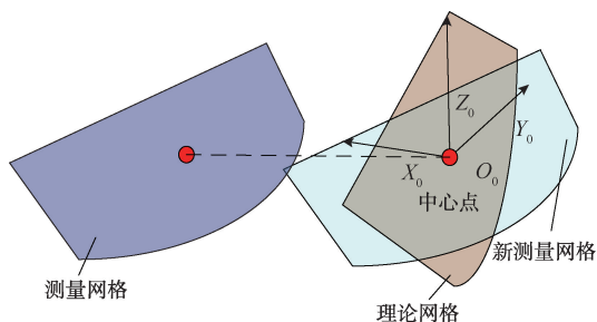
图11 齿面精匹配过程
