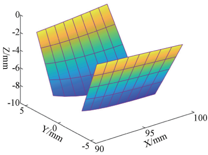
图 2 理论测量网格
