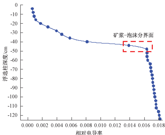
图2 矿浆相对电导率分布曲线
