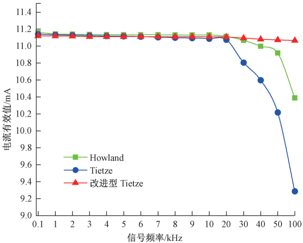
图 16 不同频率下输出电流有效值拟合 Fig. 16 Output current RMS fitting graph at different frequencies
