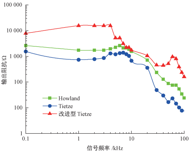
图 17 电路实际输出阻抗 Fig. 17 Actual output impedance of the circuit
