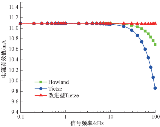
图 10 电路随频率变化的输出特性曲线
