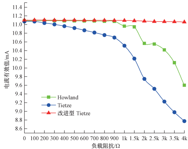
图 15 不同负载下输出电流有效值拟合 Fig. 15 Output current RMS fitting at different loads
