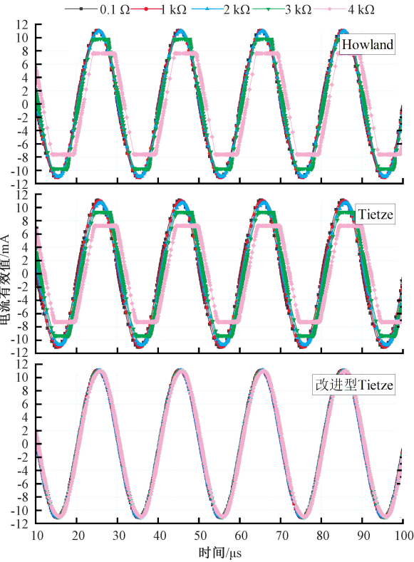
图 8 电路仿真输出波形
