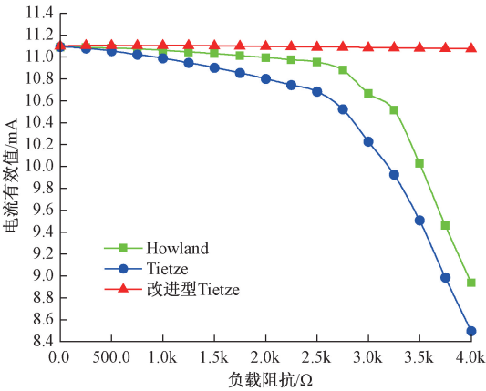
图 9 电路随负载变化的输出特性曲线
