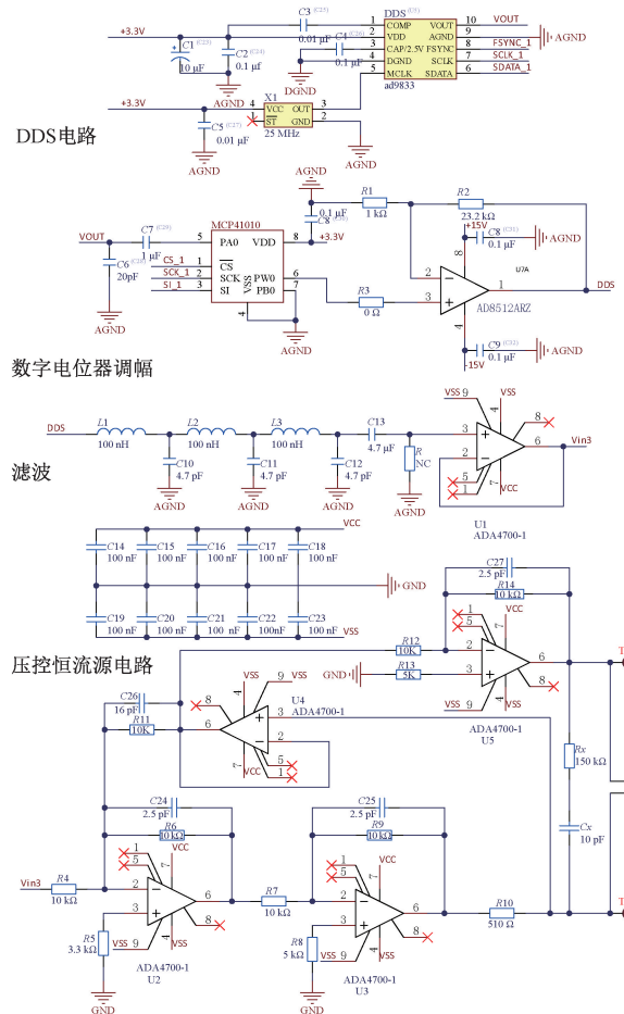
图 12 改进型 Tietze 恒流源电路原理
