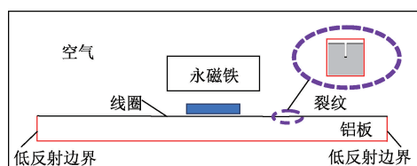
图6 EMAT 仿真模型
