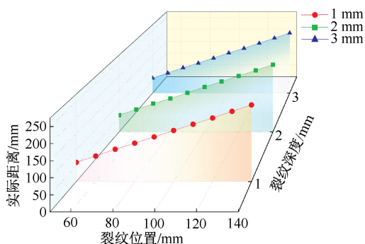
图 10 裂纹回波距离与裂纹位置关系图
