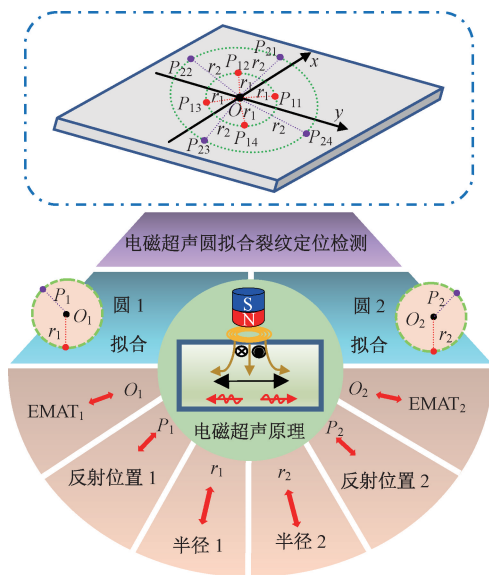
图1 电磁超声圆拟合裂纹定位方法
