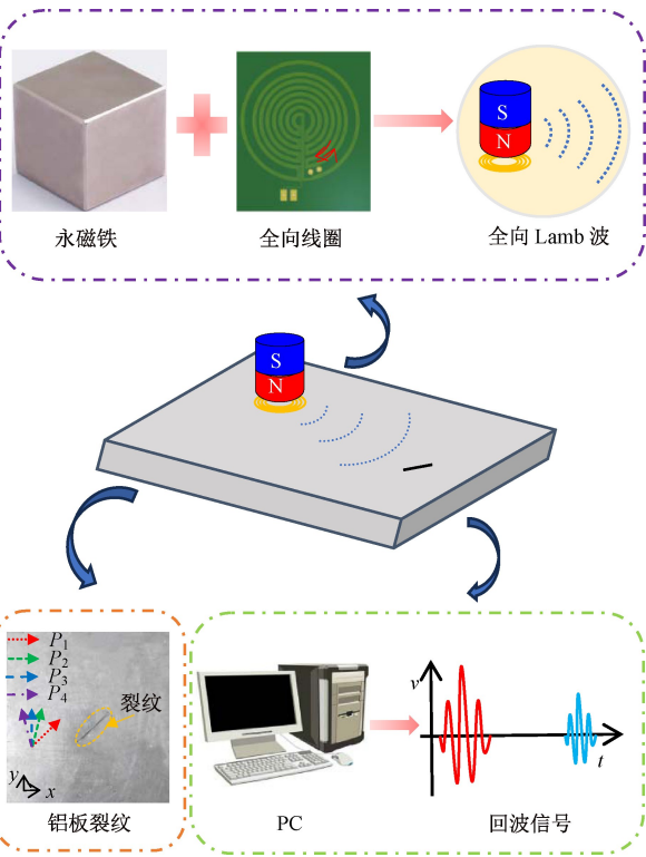
图 12 裂纹检测图
