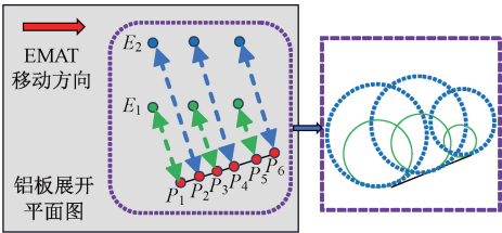
图 5 裂纹定位检测示意图
