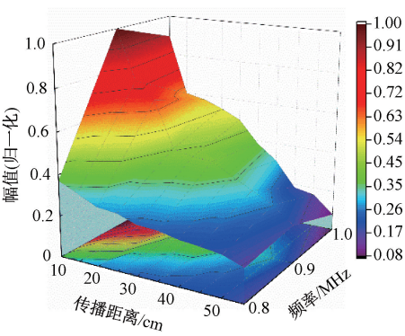
(a) 能量衰减模型 (a) Energy decay model
