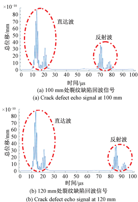
图8 不同位置裂纹缺陷回波信号图
