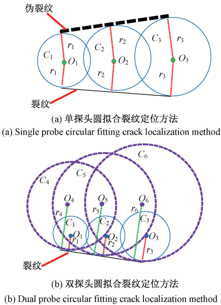
图 4 单探头及双探头圆拟合裂纹定位方法
