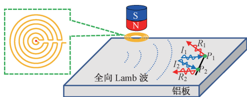
图 2 不同反射位置示意图
