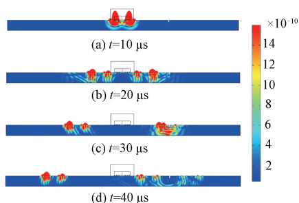
图7 裂纹缺陷反射回波位移云图
