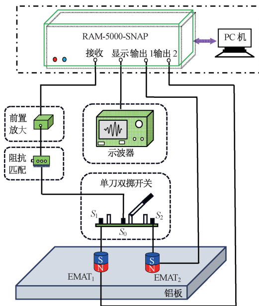
图 11 实验装置图
