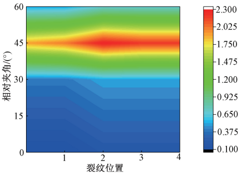
图 15 圆拟合裂纹定位误差等高线图
