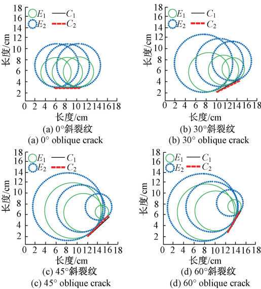
图 14 圆拟合裂纹定位检测结果图
