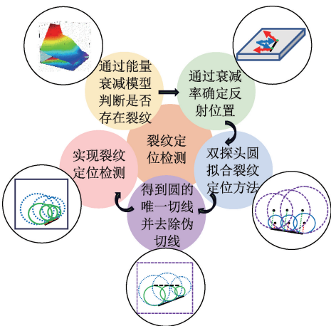
图 3 裂纹定位检测流程图
