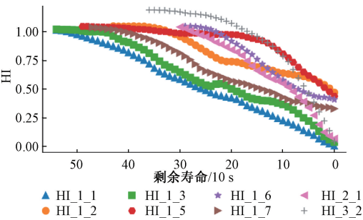
图 11 部分分解后信号的 HI 曲线
