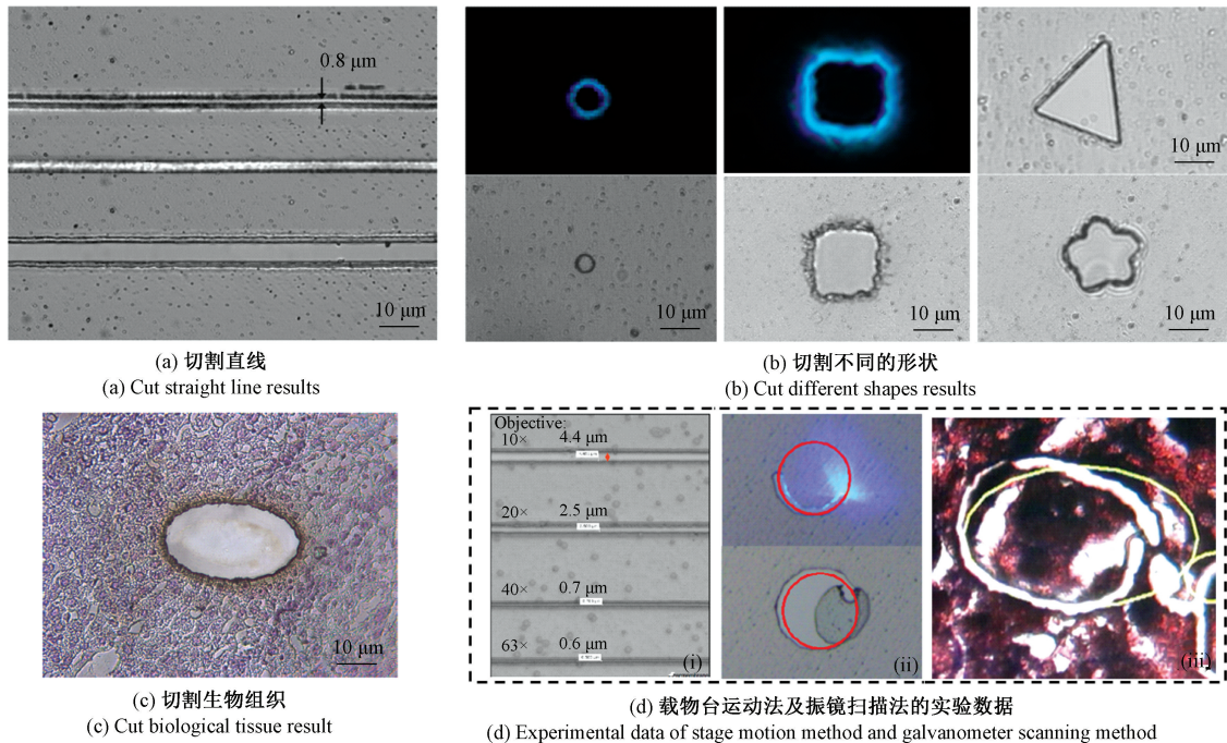
图 7 快速并行激光显微切割实验结果及比较实验数据
