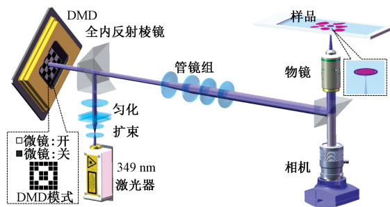
图5 实验系统示意图
