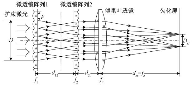
图 2 微透镜阵列匀化系统原理图
