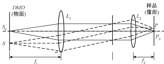
图3 基于几何光学的 DMD 投影模型
