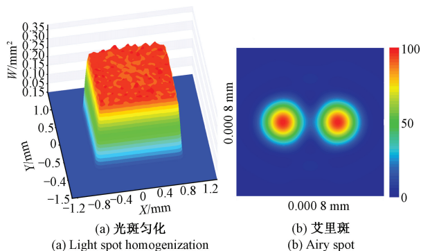
图4 匀化系统及光学分辨率仿真结果
