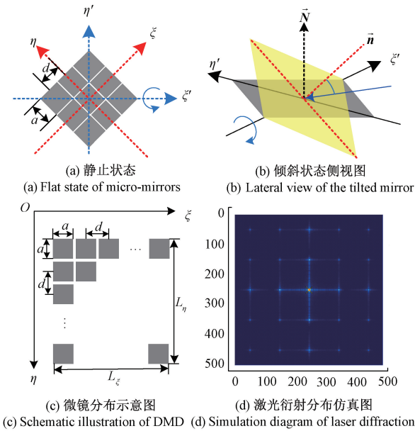
图 1 DMD 衍射特性分析
